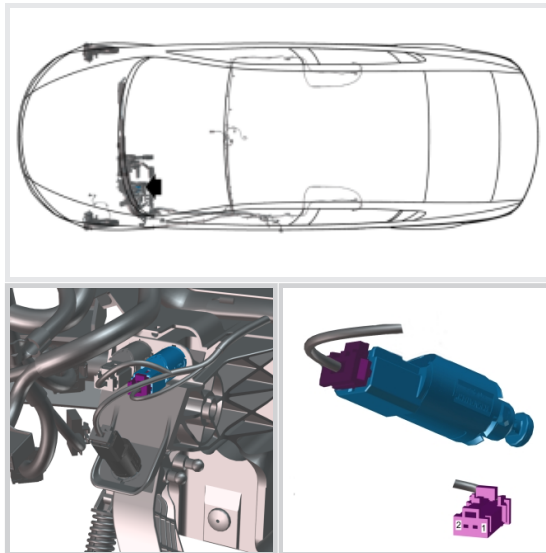
20.02.06 离合器踏板开关 - 下右 (320)
