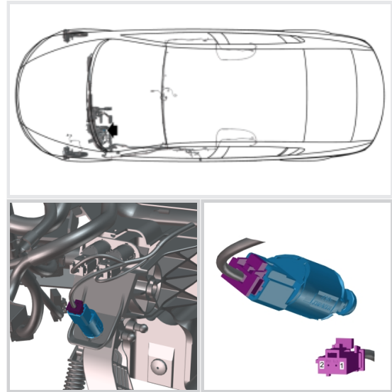
20.02.07 离合器踏板开关 - 上 (322)
