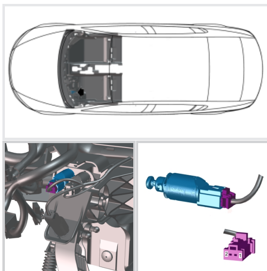
20.02.05 离合器踏板开关 - 下左 (321)
